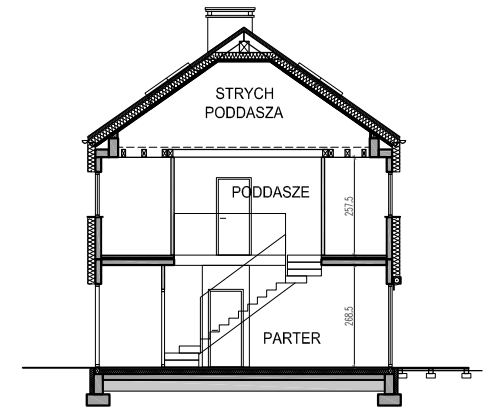
PRZEKRÓJ
