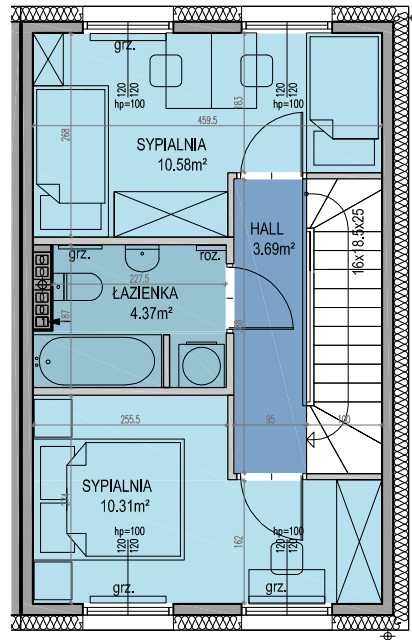
PODDASZE
