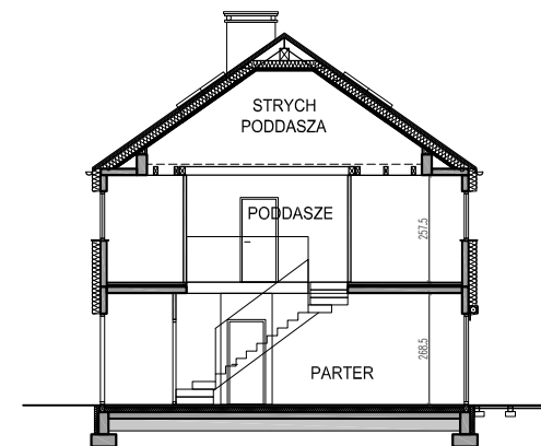
PRZEKRÓJ
