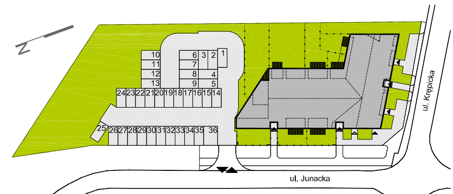
SCHEMAT ZAGOSPODAROWANIA
