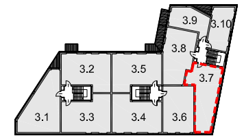
SCHEMAT KONDYGNACJI
